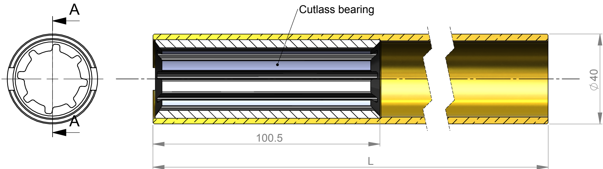
SECTION A-A
