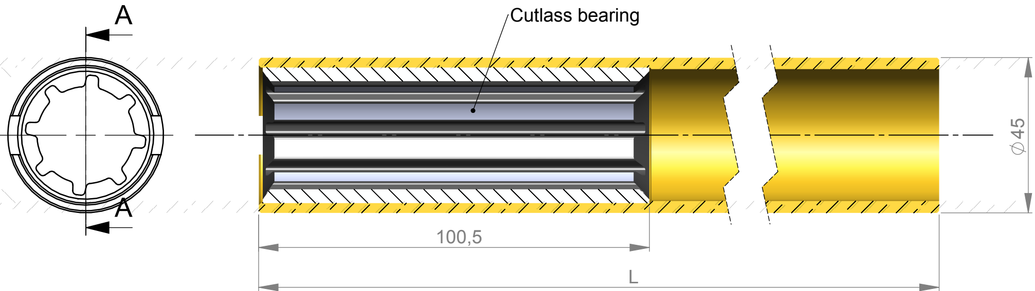
SECTION A-A
