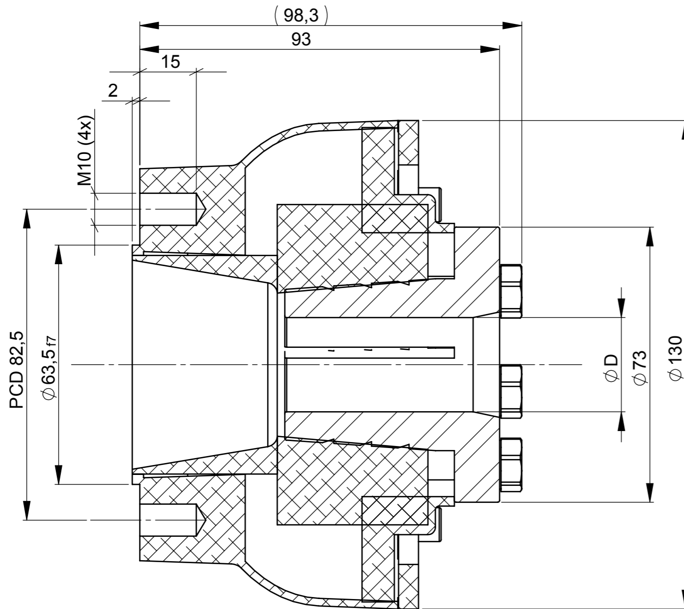
SECTION A-A SCALE 1 : 1
